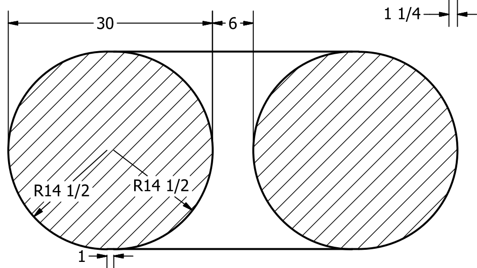
SECTION A-A SCALE 0.07 : 1
